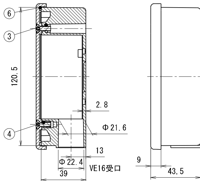
断面 A-A
